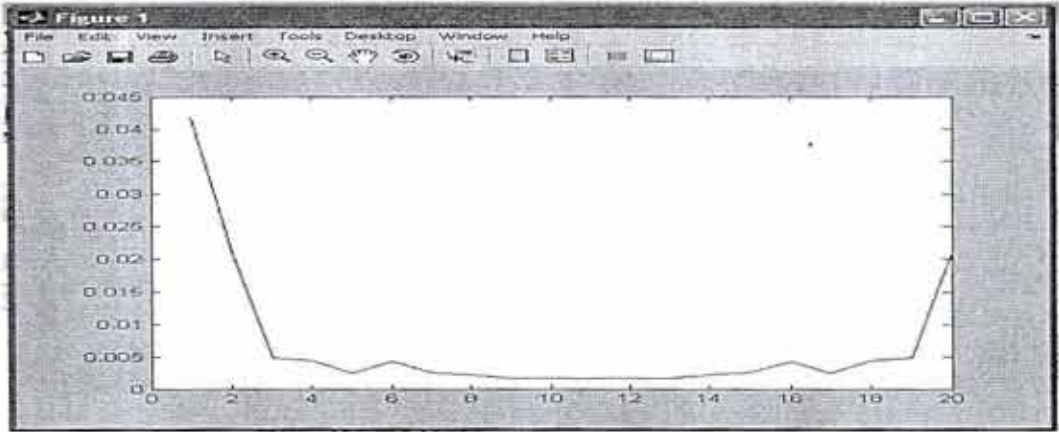
Gambar 6. Gambar Spektrum diphone 'ai'
