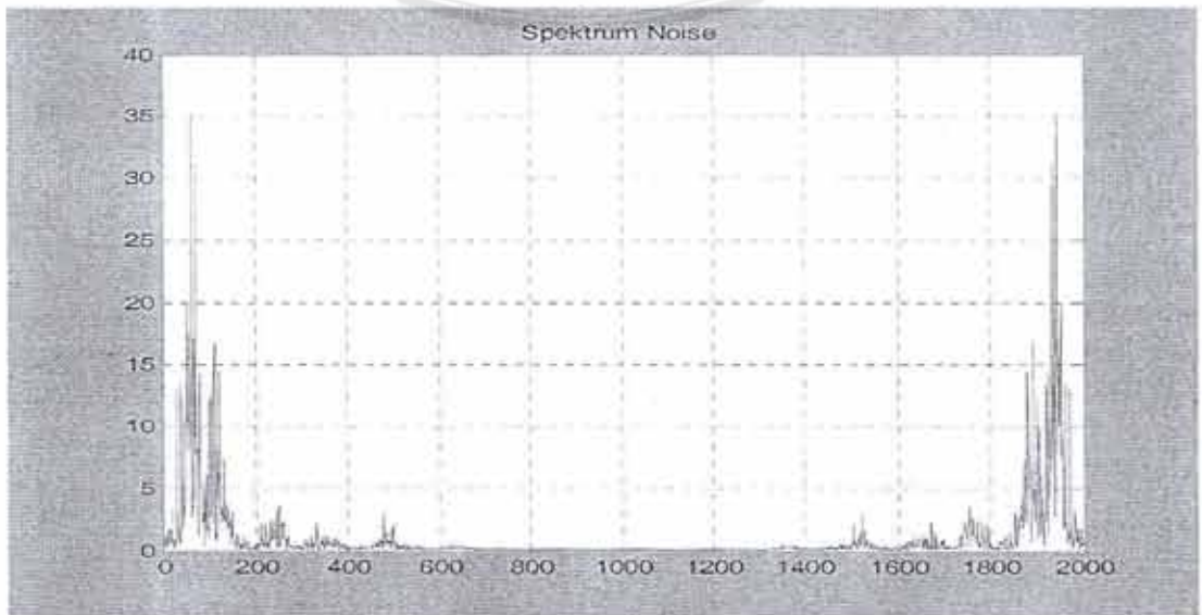
Gambar 8. Spektrum Derau
