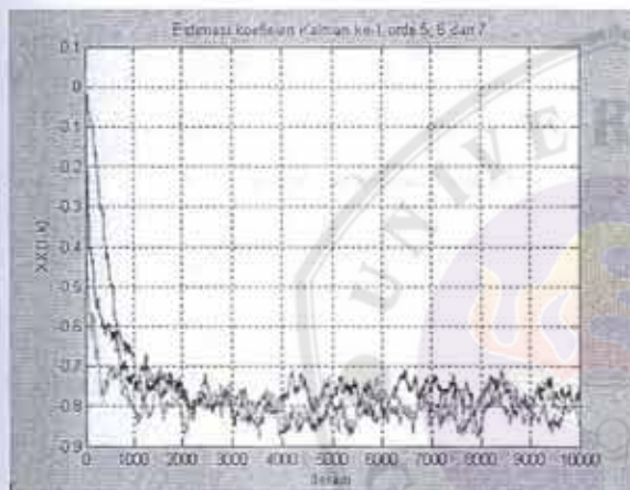
Gambar 4. Estimasi koefisien Kalman ke-1 pada orde 5, 6, dan 7
