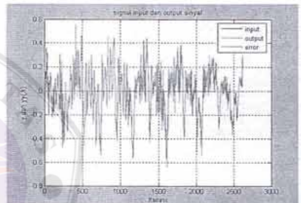
Gambar 20. Sinyal input dan output 'e' pada Q = 0,00001 dan R = 0,001
