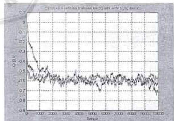
Gambar 6. Estimasi koefisien Kalman ke-3 pada orde 5, 6, dan 7
