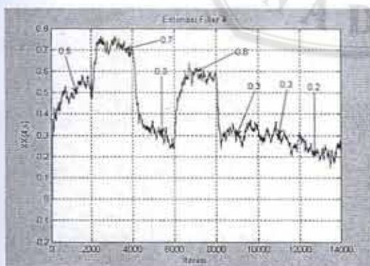
Gambar 10. Estimasi koefisien Kalman ke -4
