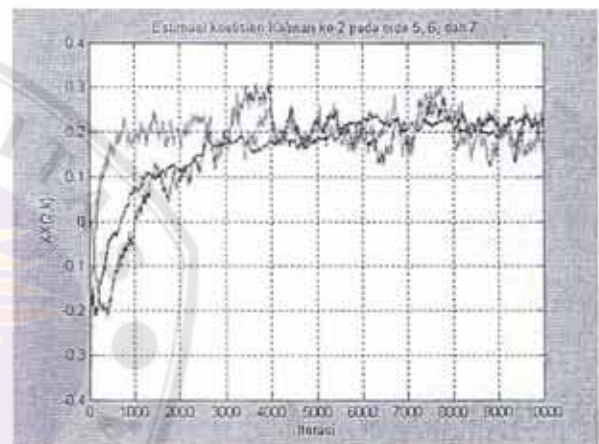
Gambar 5. Estimasi koefisien Kalman ke-2 pada orde 5, 6, dan 7
