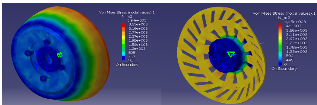
Gambar 5. Tegangan von msses pada rem cakram dan tromol
