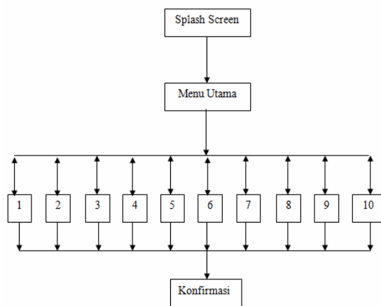
Gambar 1. Struktur Navigasi
