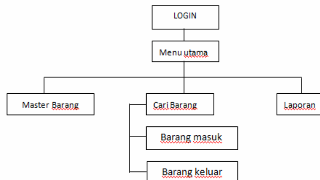
Gambar 7. Rancangan Stuktur Menu Admin
