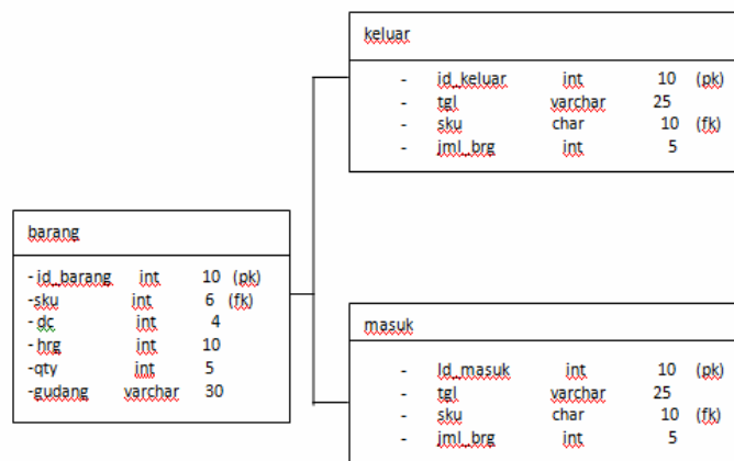
Gambar 6. Rancangan Basis Data Fisikal
