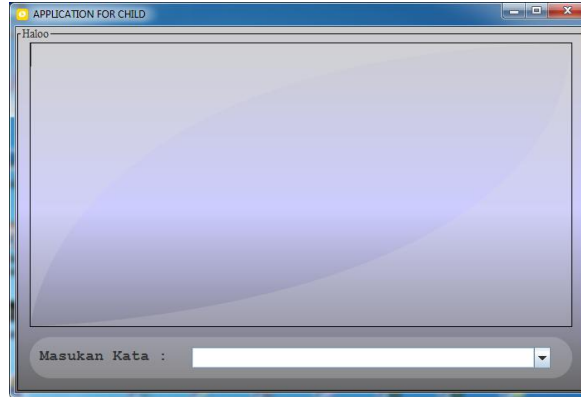
Gambar 2. Tampilan Aplikasi
